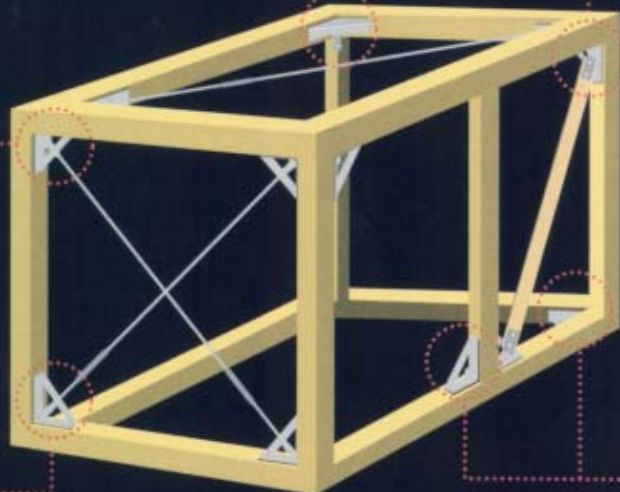
ボルイン・ワンと連結用金物で梁と柱を強固に固定
